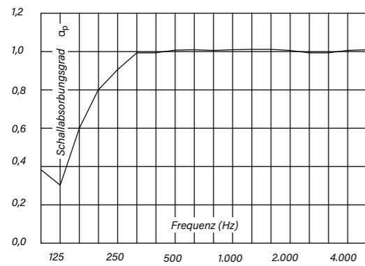
Schallabsorptionsgrad - Oktav-Mittenfrequenz
