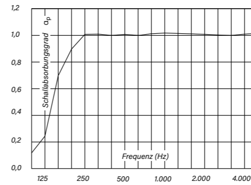
Schallabsorptionsgrad - Oktav-Mittelfrequenz
