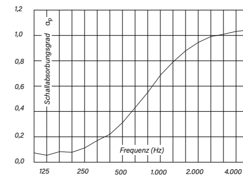
Schallabsorptionsgrad - Oktav-Mittelfrequenz
