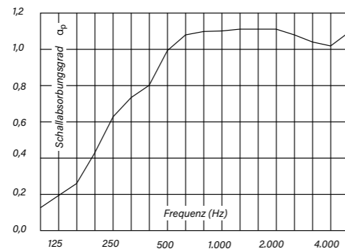
Schallabsorptionsgrad - Oktav-Mittelfrequenz (40 mm)
