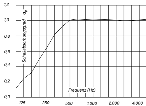
Schallabsorptionsgrad - Oktav-Mittelfrequenz
